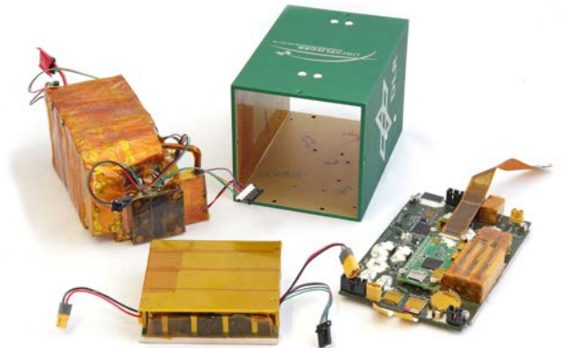
Die Größe einer Brotboxe: Auf der ISS soll EXCISS mindestens 30 Tage lang in Betrieb sein.
